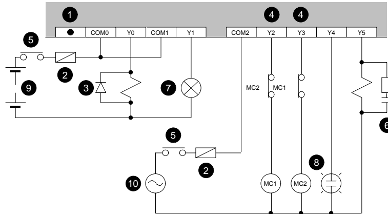
Figure 6.1 ENG ⇒ FX0-14MR-ES/UL example output wiring FRE ⇒ Exemple dn circuit de sortie pour FX 0-14MR-ES/UL GER ⇒ Beispiel einer Ausgangsbeschaltung für FX 0-14MR-ES/UL ITL ⇒ Esempio del cablaggio di uscita per FX0-14MR-ES/UL ESP ⇒ Ejemplo de una conexi de salida para FX 0-14MR-ES/UL.
