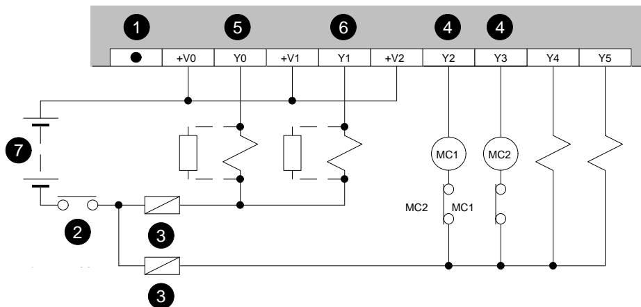
Figure 6.2 ENG ⇨ FX0-14MT-DSS example source output wiring FRE ⇨ Exemple dn branchement de sortie Source pour FX 0-14MT-DSS GER ⇨ Beispiel einer Source-Ausgangsbeschaltung für FX 0-14MT-DSS ITL ⇨ Esempio del cablaggio di uscita source per FX0-14MT-DSS ESP ⇨ Ejemplo de una conexi de salida Source para FX 0-14MT-DSS
