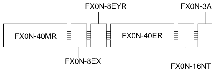
Figure: 1.7 ENG ⇨ Example FX0N system FRE ⇨ Exemple de système FX0N GER ⇨ Beispiel für ein FX0N-System ITL ⇨ Esempio del sistema FX0N ESP ⇨ Ejemplo para un sistema FX0N
